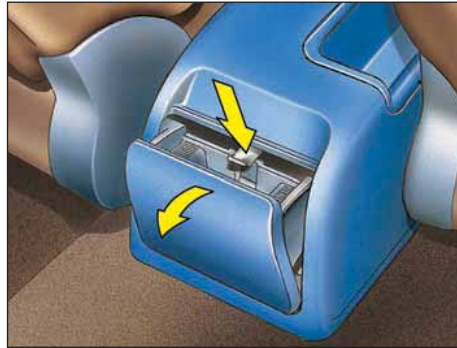
جاسیگار بها جهت خالی کردن آن، زبانه قفلی را که در زیر آن قرار دارد کشیده و آن را بلند کرده و به طرف خود بکشید. نصب جاسیگاری جاسیگاری را در جای خود قرار داده و به طور کامل به داخل فشار دهید. در روی کنسول عقب در را پایین بیاورید. جهت خالی کردن، جاسیگاری را به طرف خود کشیده و همزمان زبانه قفلی آن را به پایین فشار دهید.
