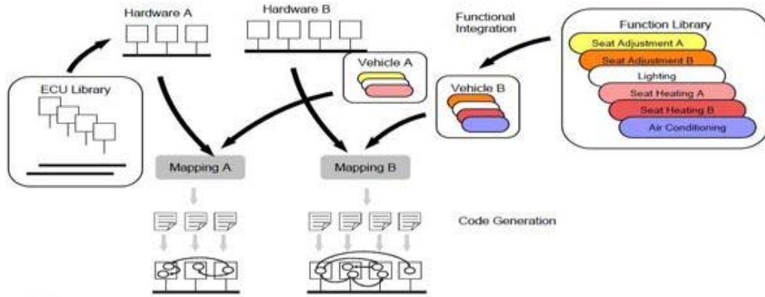
شکل ۳: اهداف AUTOSAR
