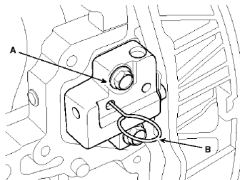
۲۲- زنجیر سفت کن هیدرولیکی (A) را باز نمایید.
