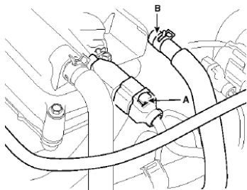
۱۲- کانکتور کوئل های جرقه (A) و لوله کنار گذر هوا (B) را نصب کنید.
