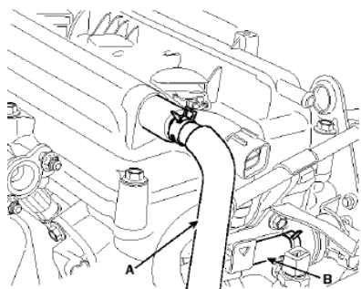
۱۱- لوله سوپاپ PCV و تخلیه بخارات بنزین PCSV را نصب کنید.
