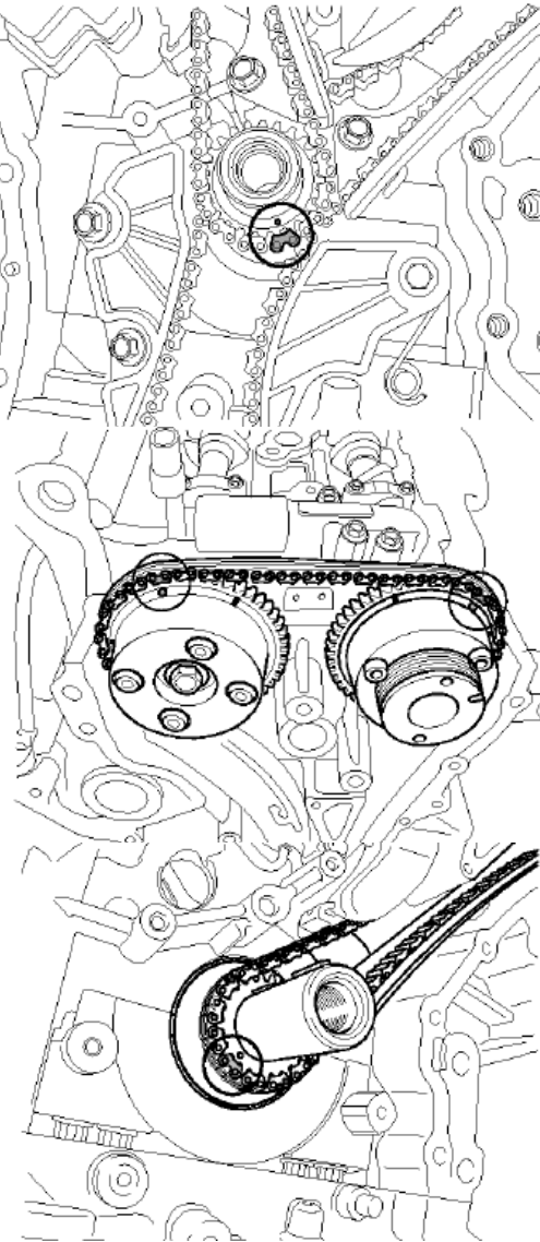
۲۳) سوپاپ OCV میل سوپاپ چپ و راست را بازنمایید.
