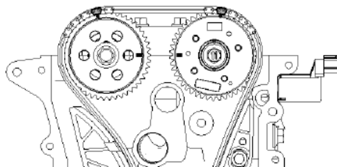
۲۲- زنجیر سفت کن هیدرولیکی (A) را باز نمایید.
