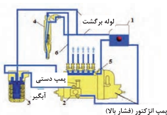
شکل ۱۳- اجزای اصلی سیستم سوخت‌رسانی دیزل مکانیکی با پمپ ردیفی
