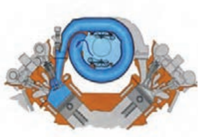
شکل ۴۱- عملکرد سیستم TUMBLE
