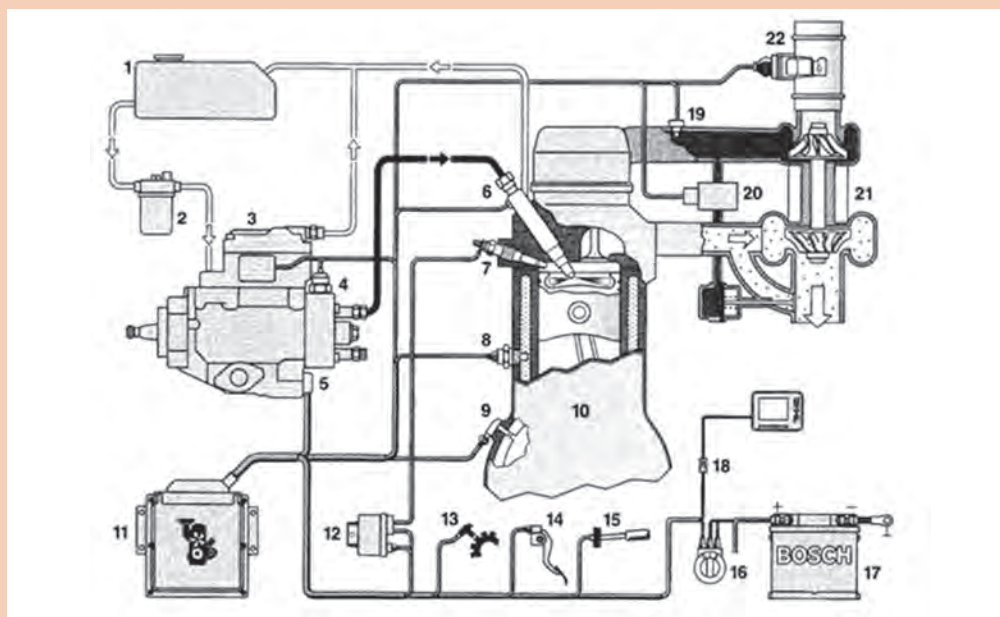
شکل ۱۲- تجهیزات مدار پمپ توزیع کننده دوار مکاترونیکی
