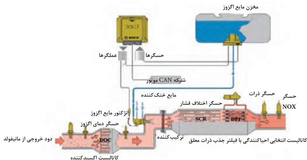
شکل ۹۱- اجزای به کار رفته در یک سیستم کنترل آلایندگی خودروهای دیزلی
