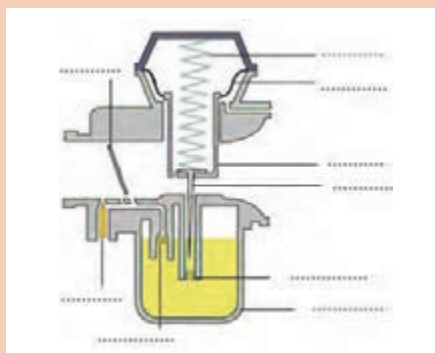
شکل ۹- کاربراتور ونتوری ثابت و متغیر
