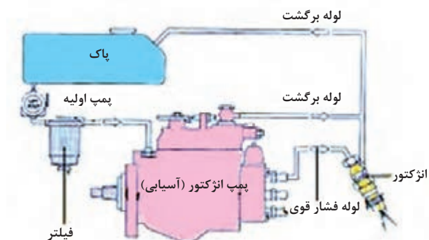
شکل ۱۴- مدار سیستم سوخت رسانی دیزل مکانیکی با پمپ انژکتور آسیابی
