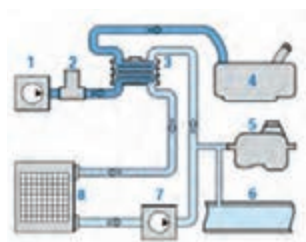
شکل ۶۵ - مدار خنک‌کاری سوخت در سیستم UIS
