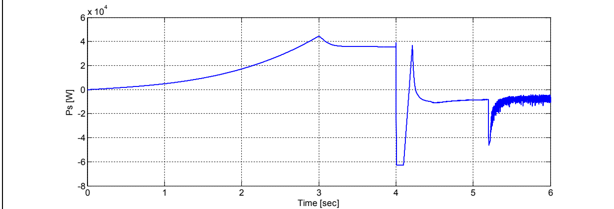
Fig. 3.68- EM generated power (negative)
